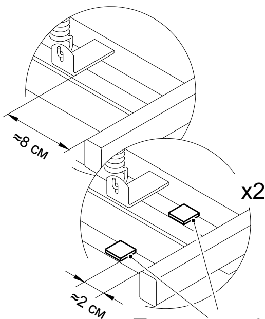
Подпятник 20x20
